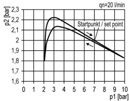
Hysterese
